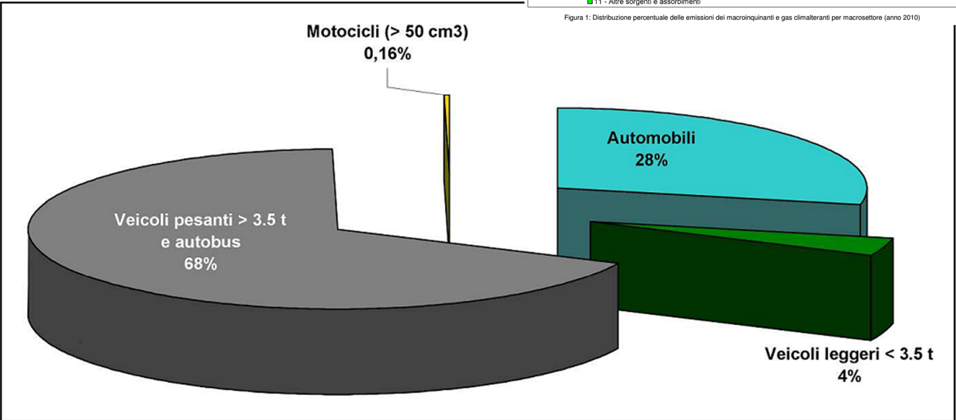
Figura 10: Quota percentuale di emissioni di NOX per tipologia di veicolo sulla A22 (2013)
